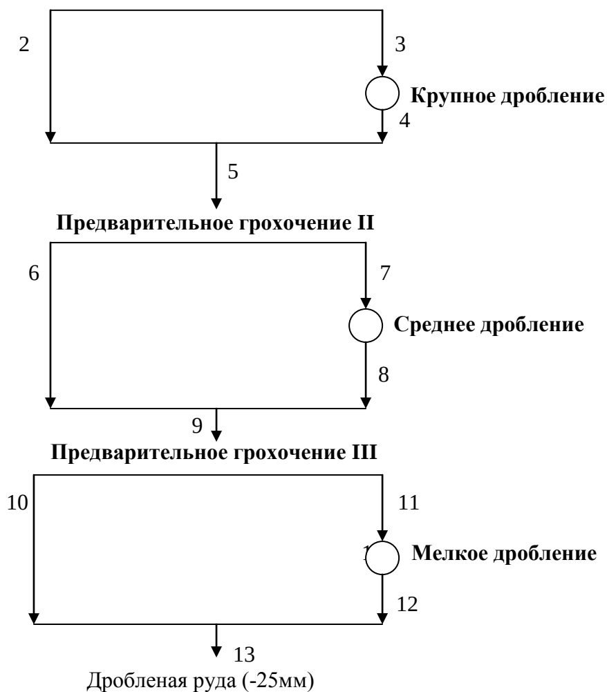
Рис. 1 Расчетная схема дробления руды
