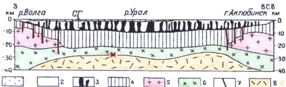
Рис. 2. Глубинный геолого-геофизический профиль через Прикаспийскую впадину. Из «Тектоники Европы» (1978).
