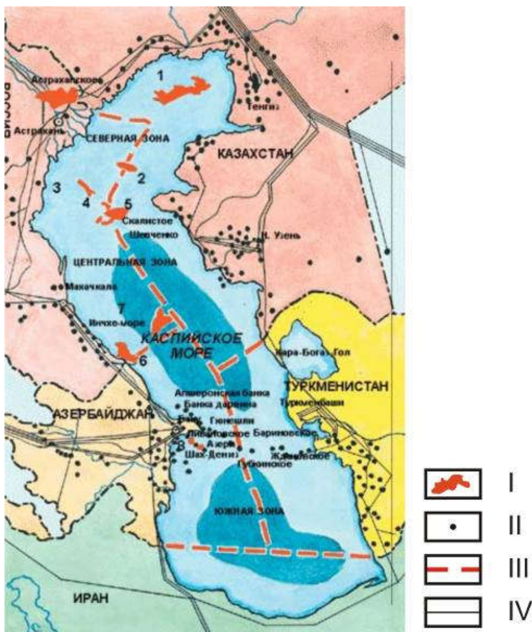
Рис.3. Каспийское море и его богатства. I – месторождения нефти и газа, открытые за последние годы и утроившие запасы Каспия:
