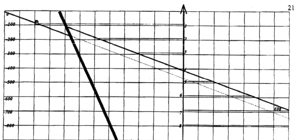
Рис.5. Шахтное поле со сбросом
