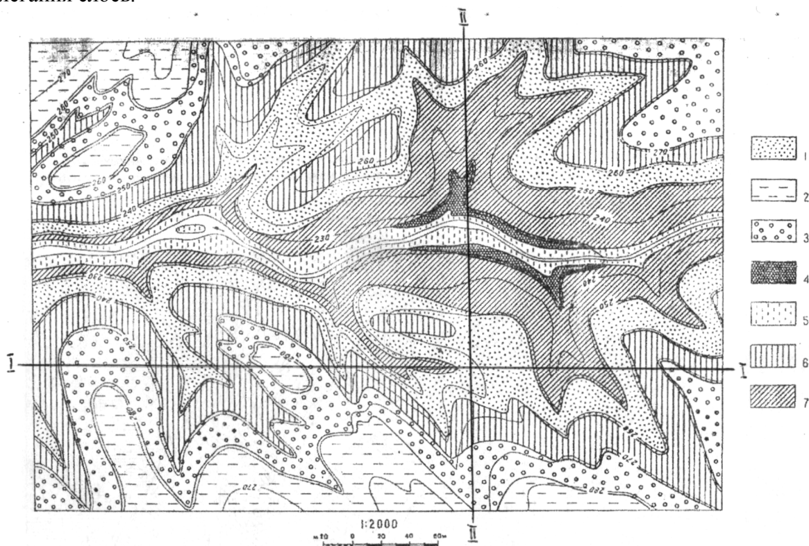
Карта 3. 1 — глауконитовые пески с линзами глин; 2 — супеси и суглинки с дресвой;
