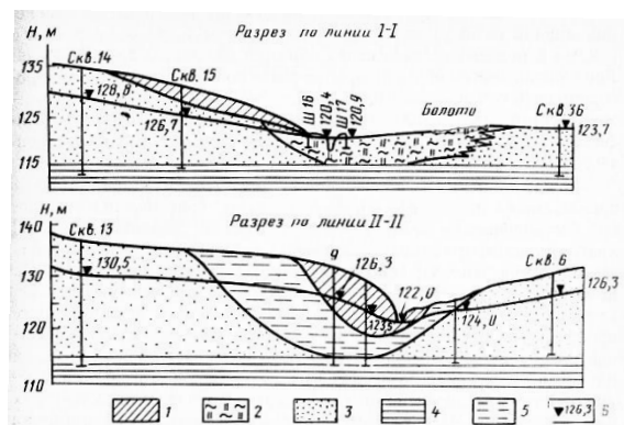
Рис. 2. Гидрогеологические разрезы по линиям I - I и II- II:
