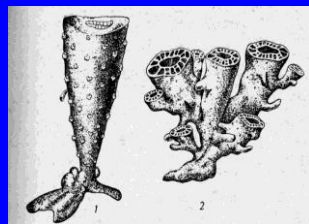
Рис. 15. Представители археоциат 1 — класс Regulares, род Tumuliolynthus (ранний кембрий); 2 — класс Irregulares, род Verthocyathus (ранний кембрий)
