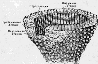
Рис. 14. Некоторые элементы строения скелета археоциат
