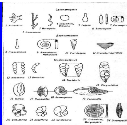
Рис. 3. Типы строения раковин фораминифер
