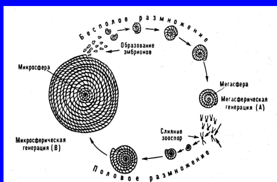
Рис. 4. Схема чередования поколений и диморфизм раковин у фораминифер на примере рода Nummulites
