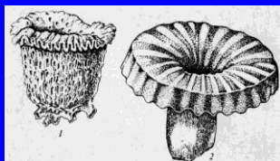
Рис. 12. Класс Hexactinellida. Роды: 1 — Ventriculites (поздний мел), 2 — Coeloptychium (поздний мел)
