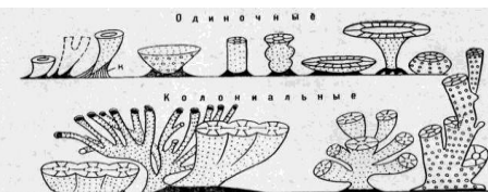
Рис. 13. Форма кубков и колоний различных археоциат (к — кабанчик прирастания)
