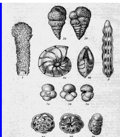
Рис. 5. Подкласс Foraminifera. Мелкие фораминиферы из отрядов Astrorhizida (1), Textulariida (2), Nodosariida (3-4), Rotaliida (5-6). Роды: 1 — Hyperammina (ранний палеозой-ныне), 2 a, б — Textularia (юра-ныне); 3 — Nodosaria (пермь-ныне), 4 a, б — Leniculina (триас-ныне), 5 a-в — Globigerina (юра-ныне), 6 a - в — Sireblus (миоцен-ныне)
