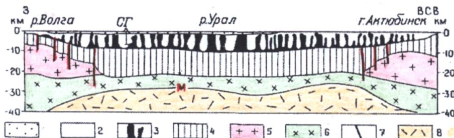
Рисунок 1. Глубинный геолого-геофизический профиль через Прикаспийскую впадину. Из «Тектоники Европы» (1978).
