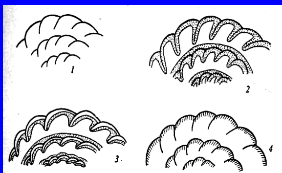
Рис. 6. Типы строения стенок раковины фузулинид 1 — однослойная, 2 — трехслойная, 3 — четырехслойная, 4 — двухслойная
