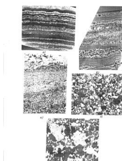
Рисунок 1.3. Морфологические особенности «пиритовых ритмитов» (а, б) и их внутреннее строение (в, г, д).
