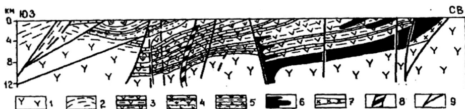
Рисунок 2.7. Геологический разрез через Имандра-Варзугскую впадину (по В.Г.
