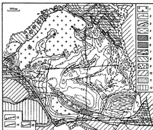
Рисунок 2.2. Схематическая карта рельефа поверхности фундамента Восточно-Европейской платформы и смежных метаплаตฟอร์มных областей. Составлена по тектонической карте Европы масштаба 1 : 10 000 и другим материалам.
