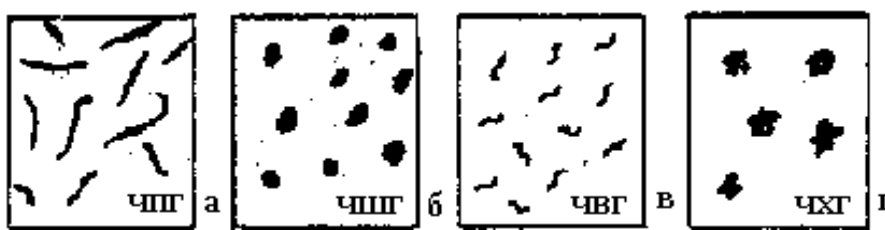
Рис. 5. Структурная диаграмма чугунов (толщина стенки отливки постоянная)
