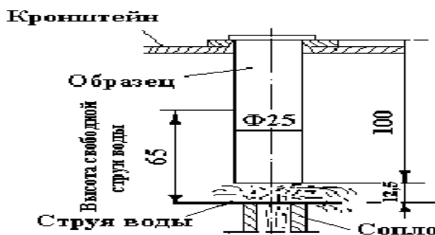
Рис. 16. Схема установки образца при испытании на прокаливаемость методом торцевой закалки
