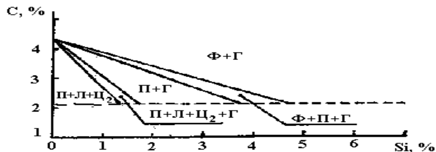
Рис. 5. Структурная диаграмма чугунов (толщина стенки отливки постоянная)
