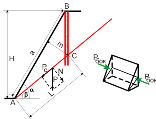
Рис. 2 – Схема расчета устойчивости борта карьера 1 – структурные нарушения I порядка; 2 – структурные нарушения II порядка
