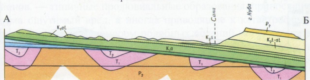
Рисунок 4. Геологическая карта и разрез с субгоризонтальным залеганием слоев более молодых кайнозойских горных пород.
