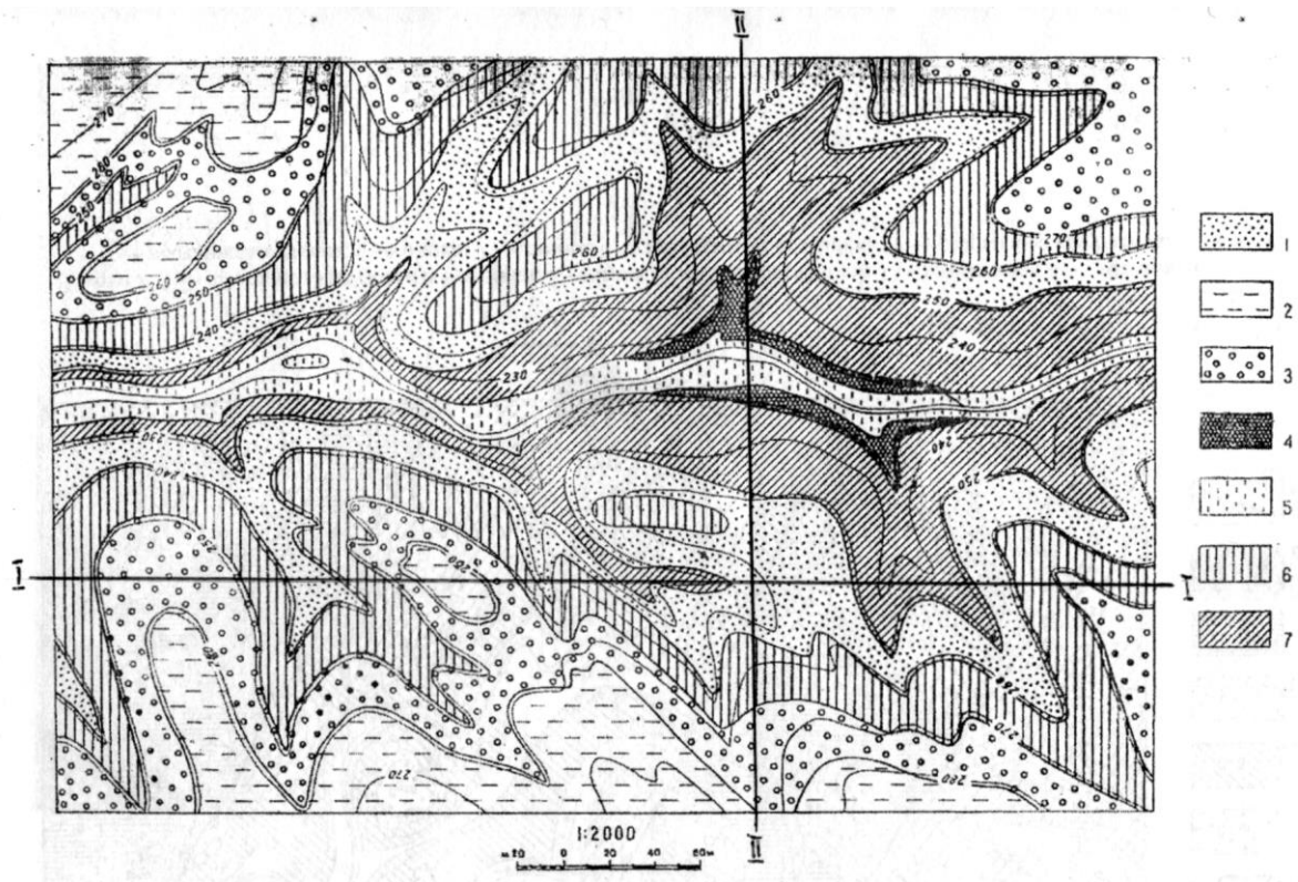
Карта 2. 1 — глауконитовые пески с линзами глин; 2 — супеси и суглинки с дресвой; 3 — галечники с линзами суглинков; 4 — органогенные известняки; 5 — аллювиальные пески и супеси с галькой; 6 — глины с прослоями песков; 7 — пелитоморфные известняки. Нормальная последовательность знаков в легенде не сохранена.
