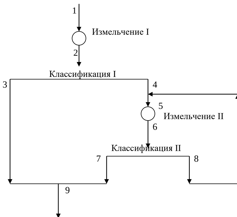
Рис. 2 Расчетная схема измельчения руды
