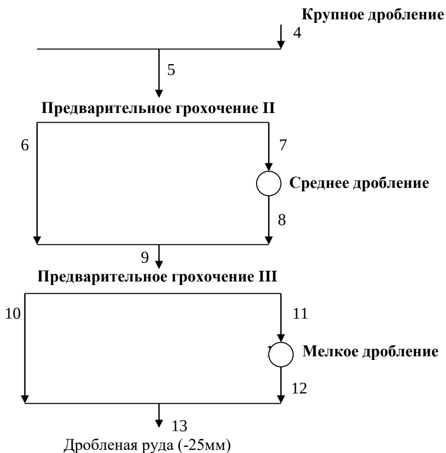
Рис. 1 Расчетная схема дробления руды
