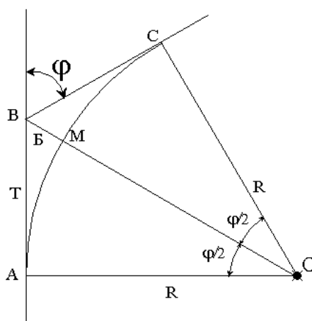
Рисунок 2. Пояснительная схема к составлению проекта по разбивке кривой.
