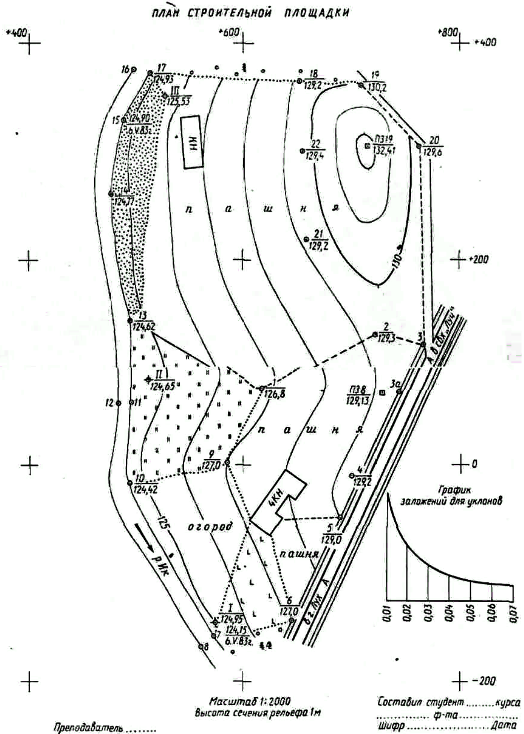
Рис. 9. Образец оформления составленного топографического плана
