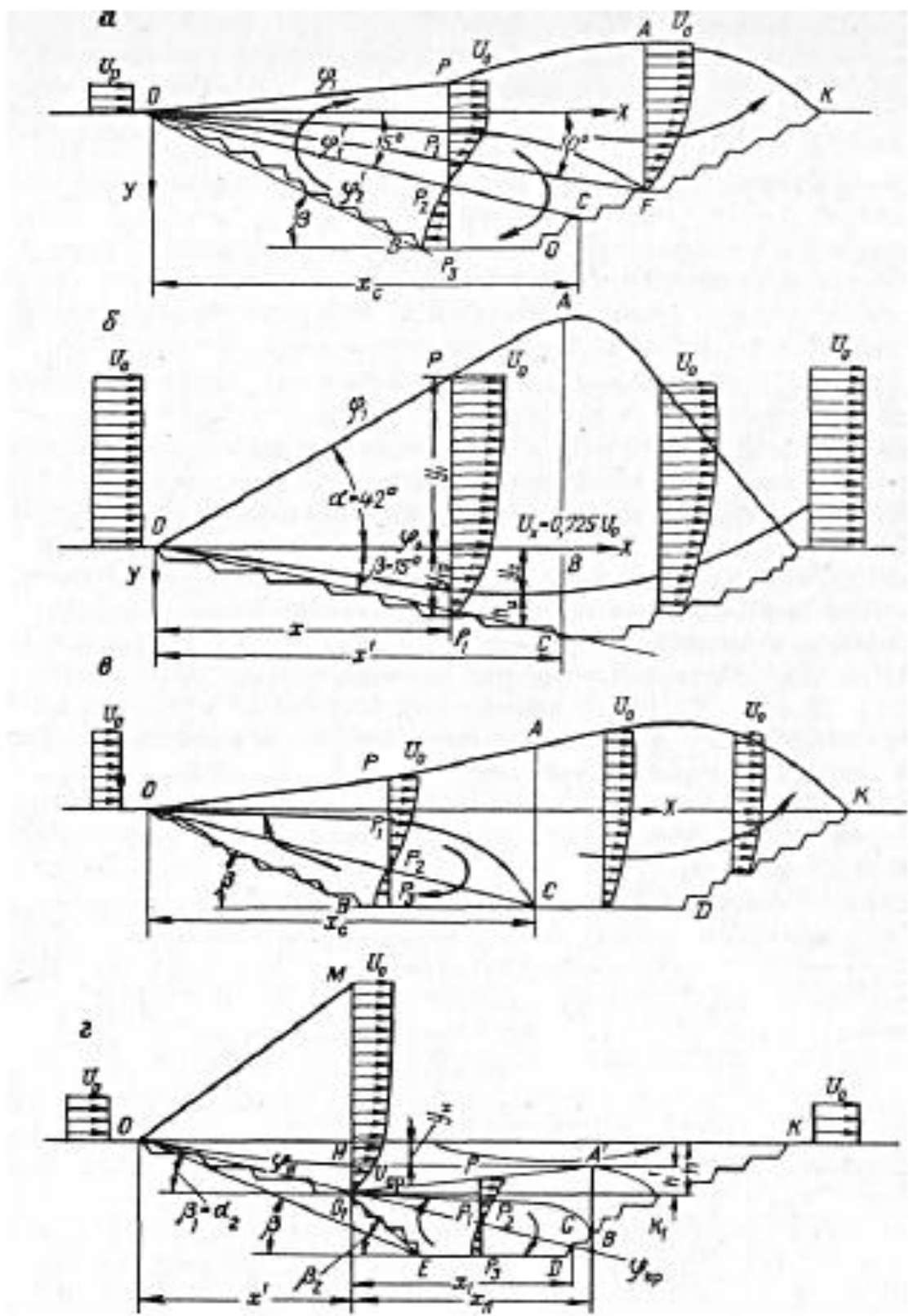
Рис. 1. Структура воздушного потока при: а – рециркуляционной; б – прямоточной; в – рециркуляционно-прямоточной; г – прямоточно-рециркуляционной схемах естественного проветривания карьера
