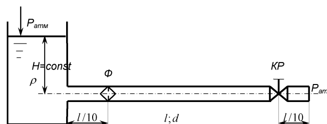
Рисунок 1.1 – Схема системы, состоящей из гидробака и трубы постоянного сечения.
