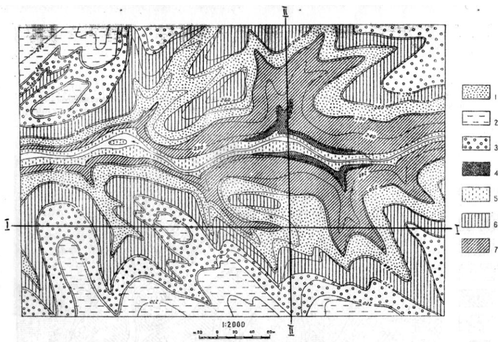
Карта 3. Геологическая карта с субгоризонтальным залеганием пластов.
