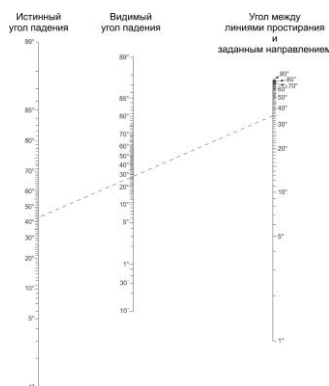
Рис. 8. Номограмма для определения видимого угла падения в сечении не перпендикулярном простиранию пласта.
