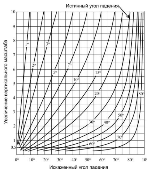
Рис. 9. Номограмма для определения угла падения слоя при увеличении вертикального масштаба разреза.
