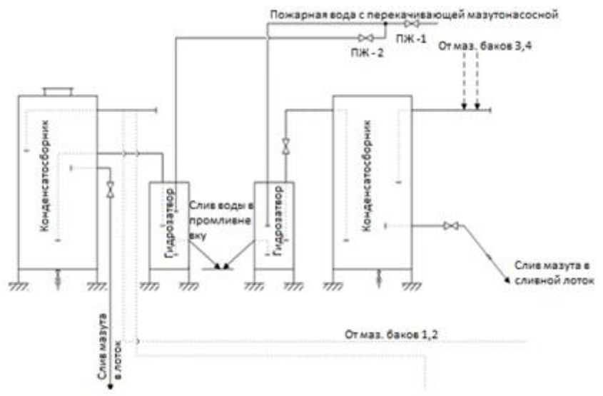
Рисунок 1. Действующая схема отвода пароводяной смеси
