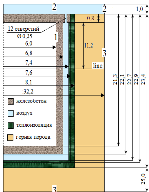
Рисунок. Модель реакторной выработки подземной АСММ (размеры указаны в м): 1 – поверхность ограждающей конструкции реакторного отделения;
